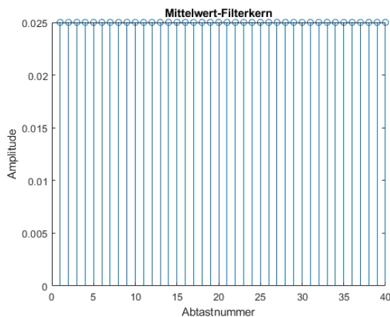
Abb. 2: Filterkern Mittelwert-Filter
