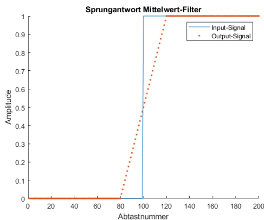
Abb. 3: Sprungantwort Mittelwert-Filter
