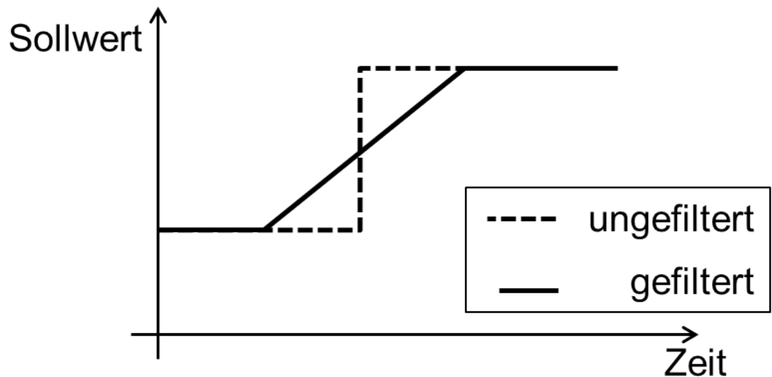
Abb. 1: Sprungantwort Achssollwertfilter
