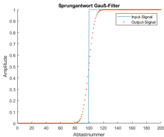
Abb. 5: Sprungantwort Gauß-Filter
