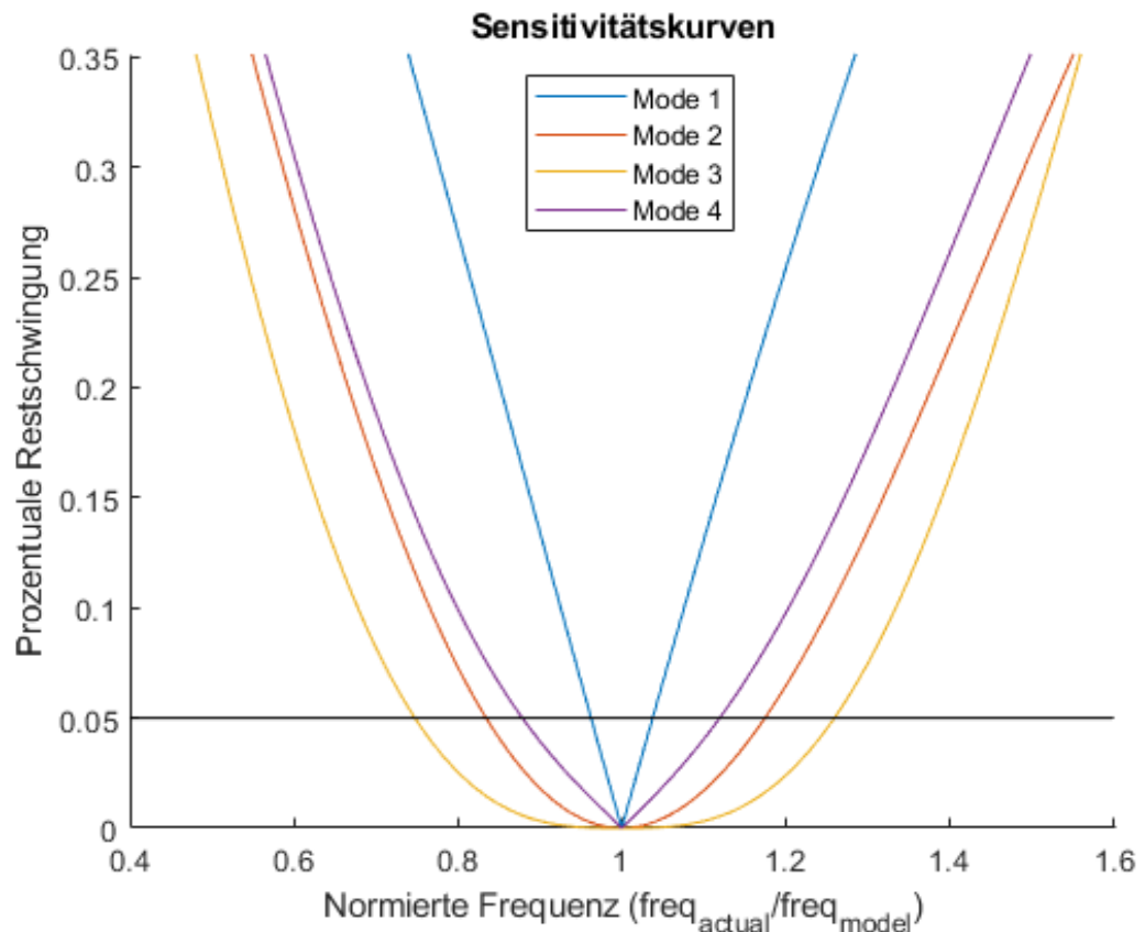
Abb. 2: Robustheitsbereiche für eine Restschwingung von 5% bei damping=0.1
