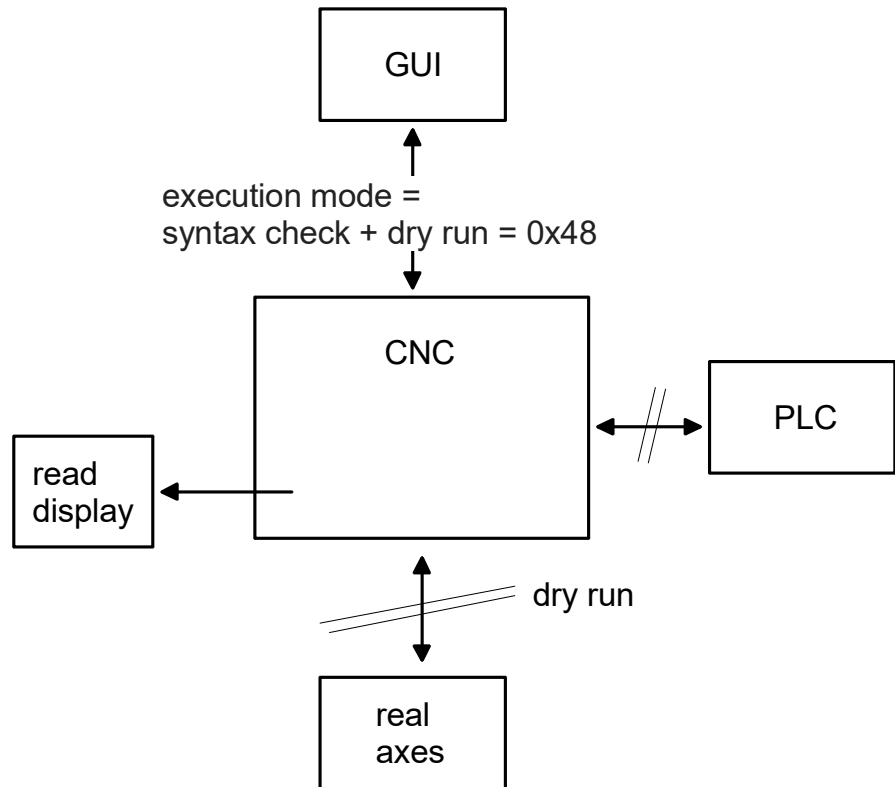
Abb. 1: Syntaxcheck ohne Antriebe
