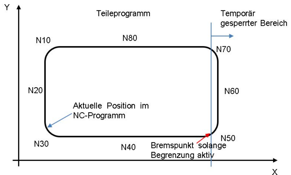
Abb. 1: Begrenzungsdarstellung, Bremspunkt zwischen N40 und N50
